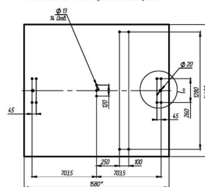
Монтажная схема установки QL-10
