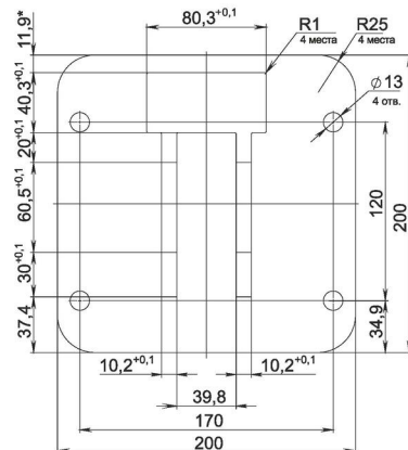
Основание стойки ограждения T-10
