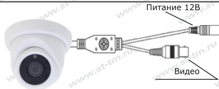
Рис.1 Схема подключения
